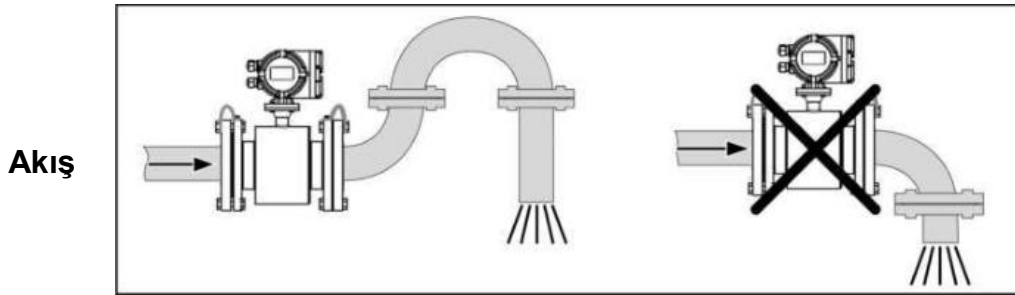
Şekil-11 Çıkışı Açık Bir Boru Hattında Sensör'ün Yatay Bağlantısı
