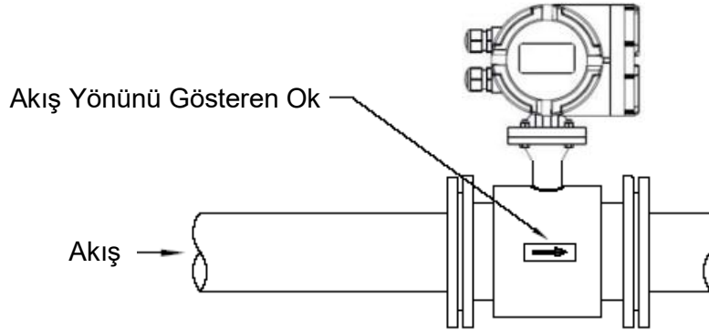
Şekil-18 Akış Yönü
