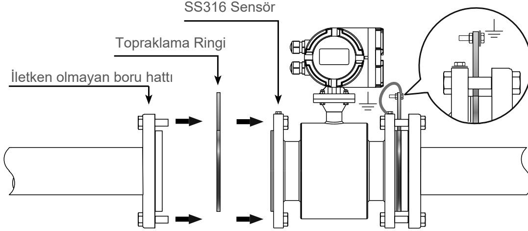
Şekil-22 İletken Olmayan Boruda Topraklama Ringleriyle Debimetrenin Topraklanması
