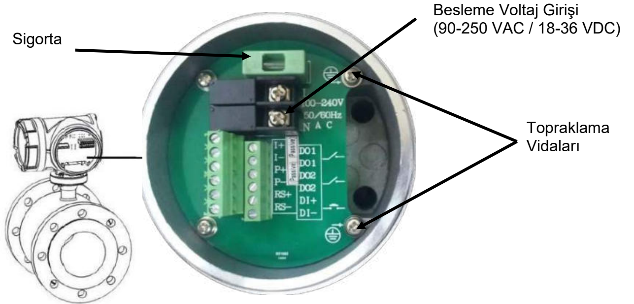
Şekil-24 Besleme Kablo Bağlantıları.
