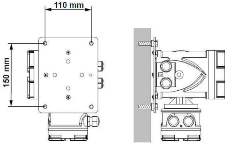
Şekil-4 Duvar Montajlı Remote Gösterge Montajı ve Boyutları
