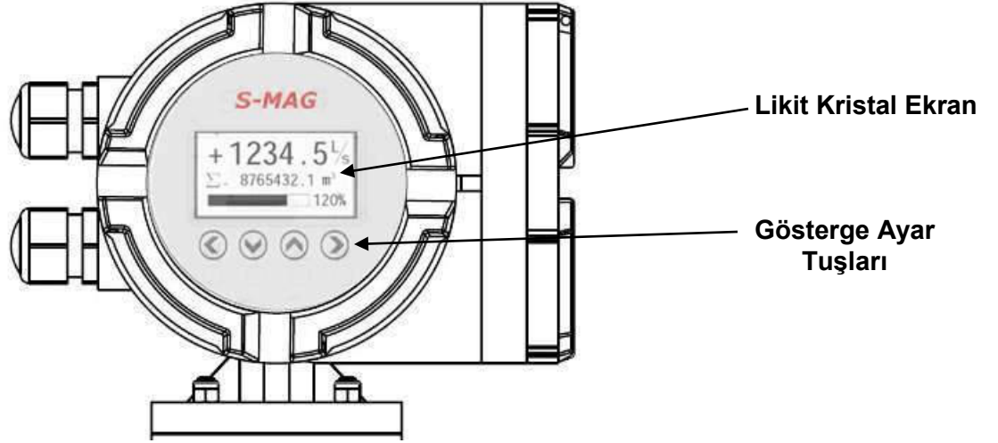
Şekil-28 S-MAG 100 Model Debimetrenin Göstergesi
