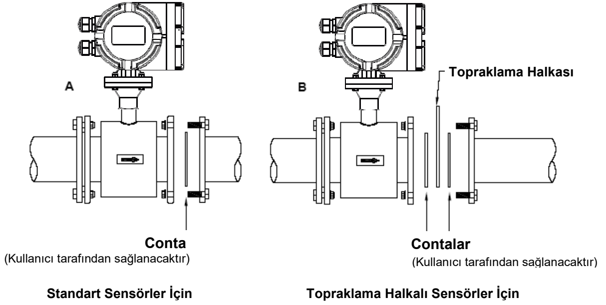
Şekil-19 Flanş Contaları
