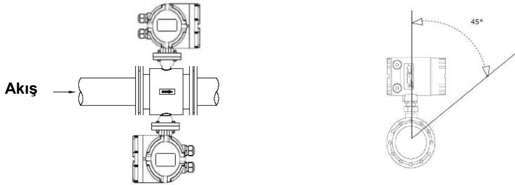
Şekil-10 Sensör'ün Boru Hattına Yatay Bağlanması
