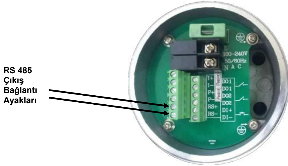
Şekil-27 RS485 Bağlantıları
