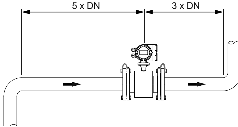
Şekil-7 Debimetreden önce ve sonra Düz Boru Mesafesi
