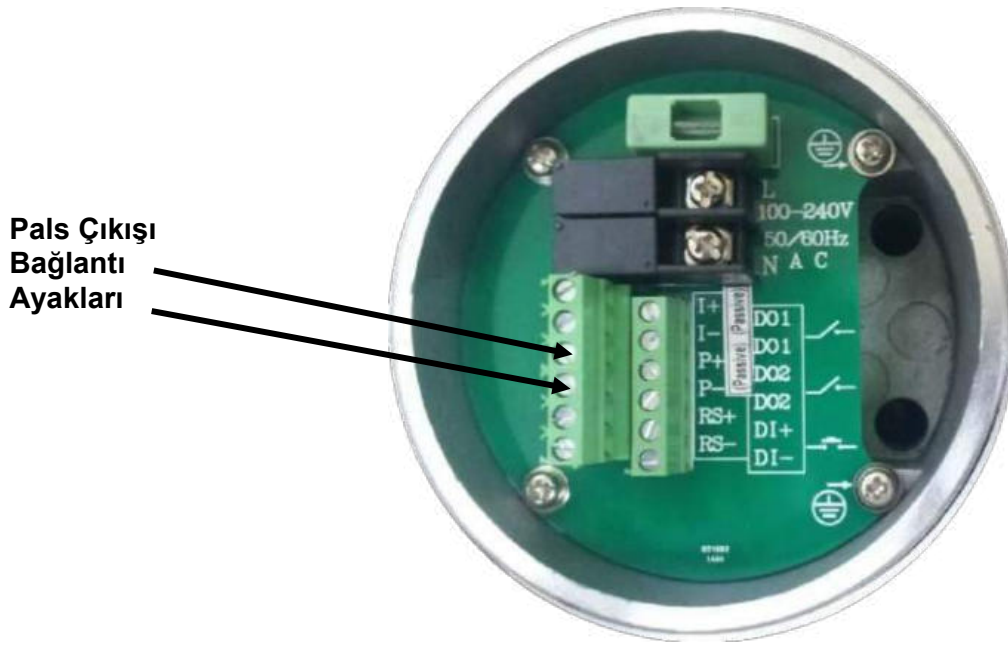
Şekil-26 Pals Çıkış Bağlantıları
