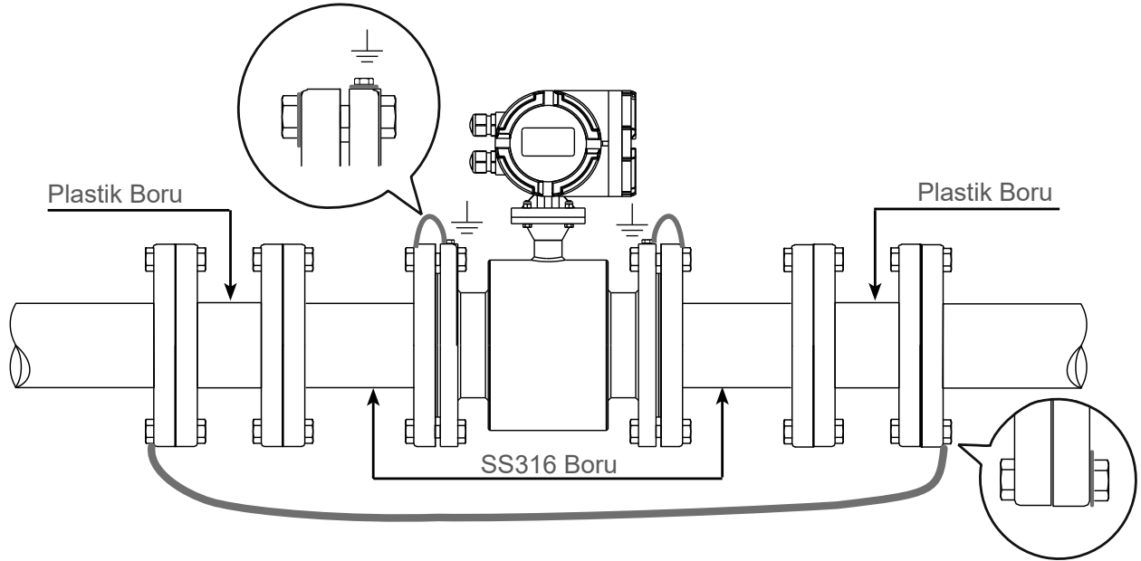
Şekil-23 Katodik Korumalı Boruda Debimetrenin Topraklanması
