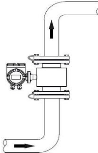
Şekil-8 Sensör'ün Dikey Bağlantı Şekli
