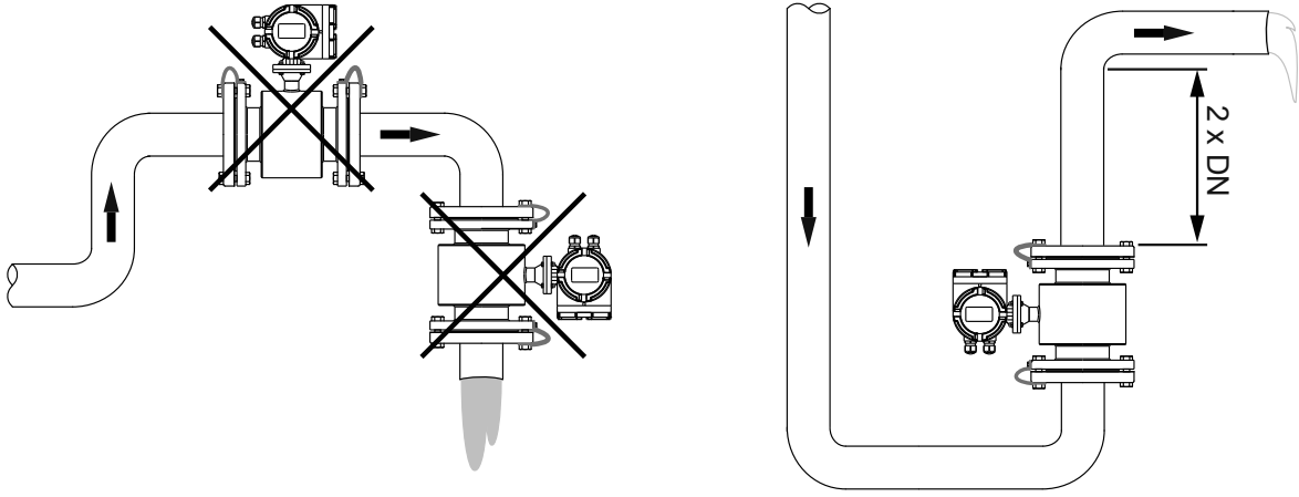
Şekil-9 Yukarı ve Aşağı Yönde Giden Bir Boru Hattında Sensör'ün Bağlantısı
