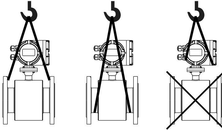
Şekil-6 Sensör'ün Taşıma Şekli
