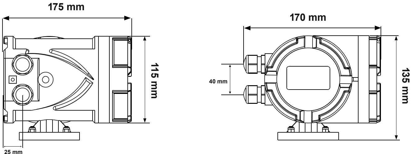
Şekil-5 S-MAG 100 Gösterge Boyutları
