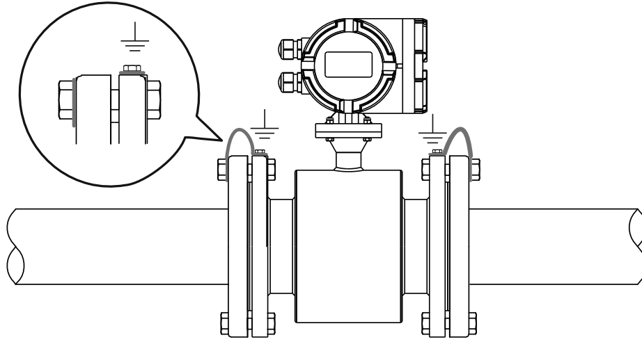
Şekil-21 İletken Bir Boruda Debimetrenin Topraklanması.
